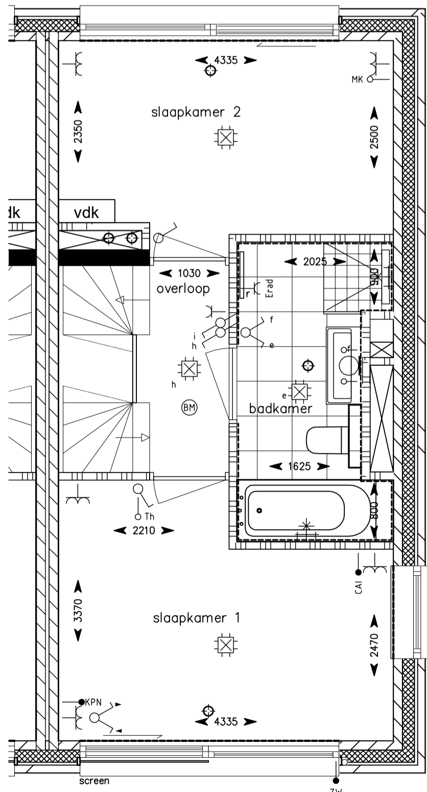
2e verdieping
