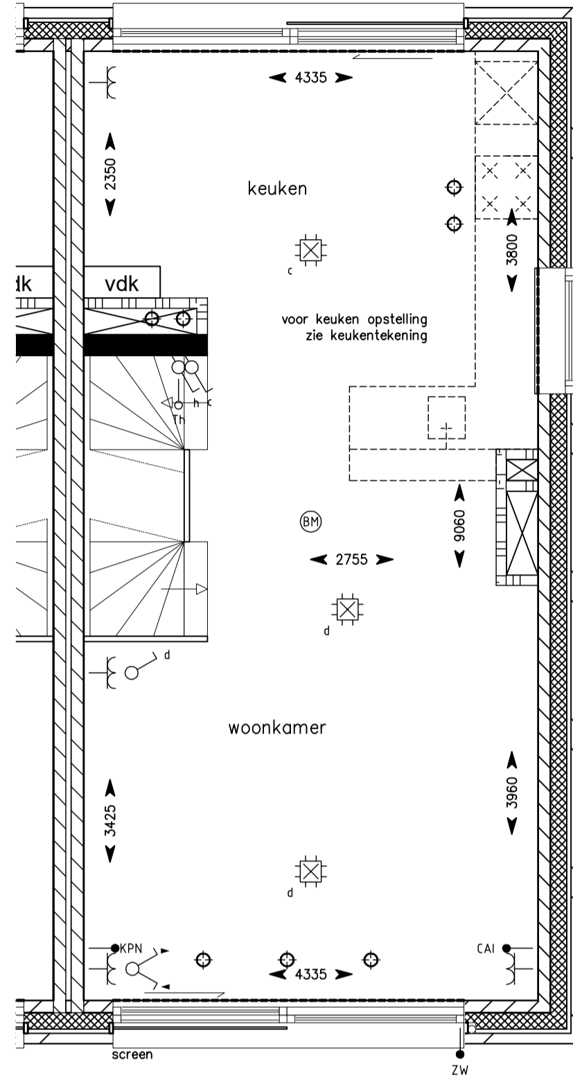
1e verdieping
