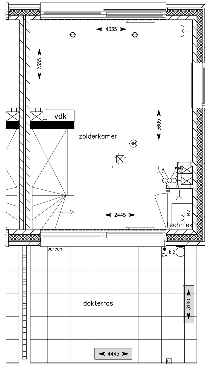
3e verdieping
