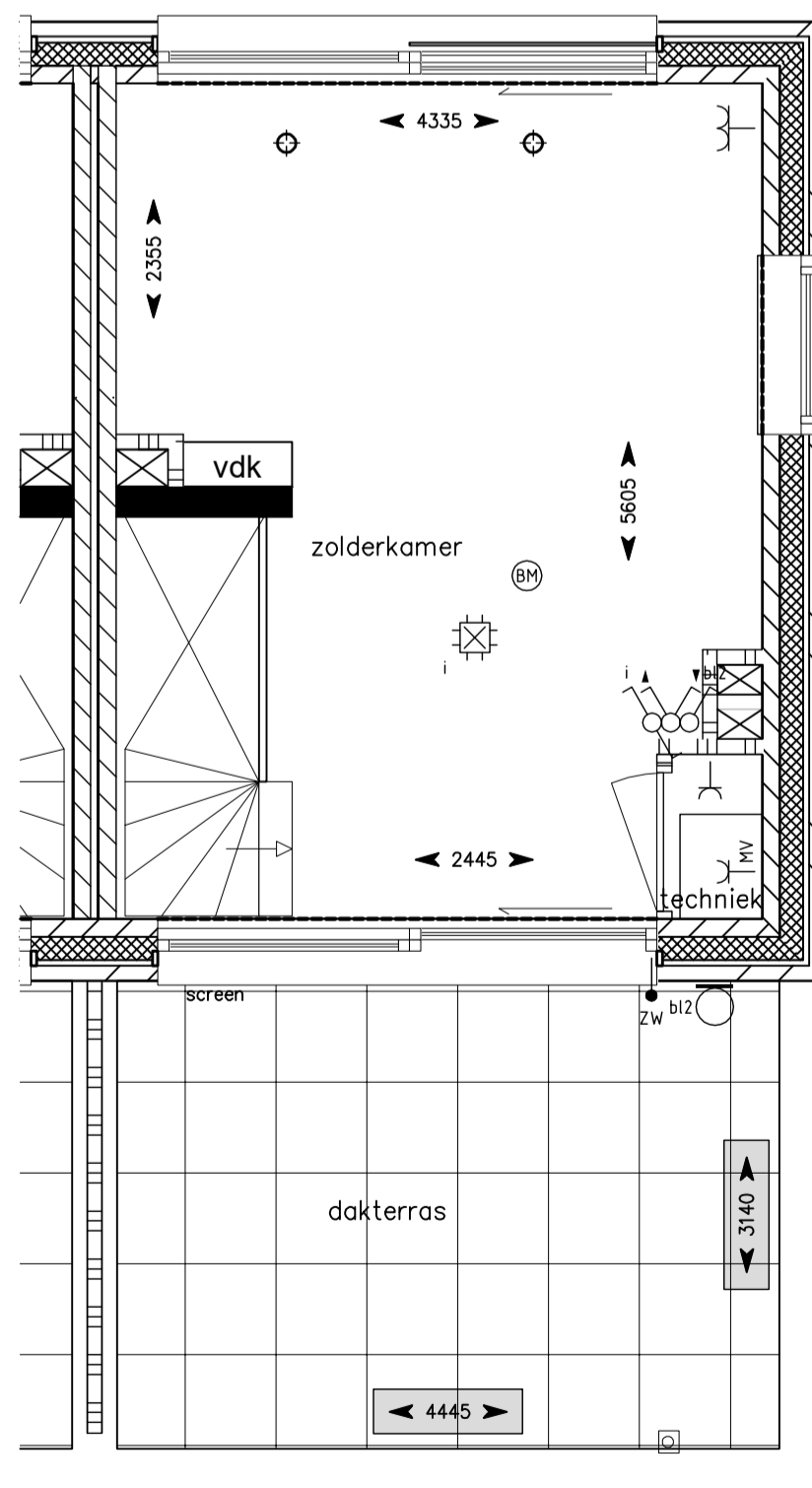
3e verdieping
