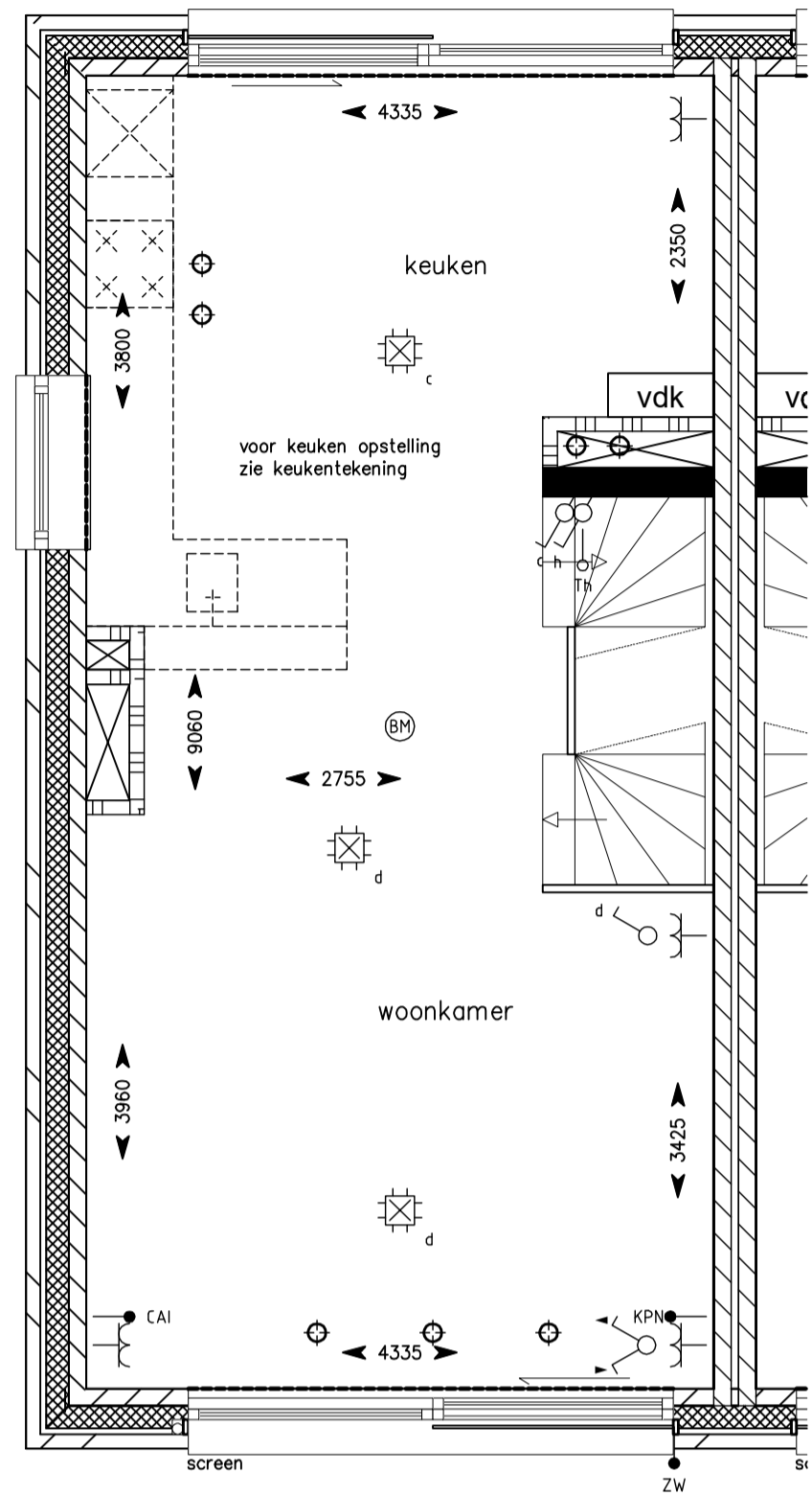
1e verdieping
