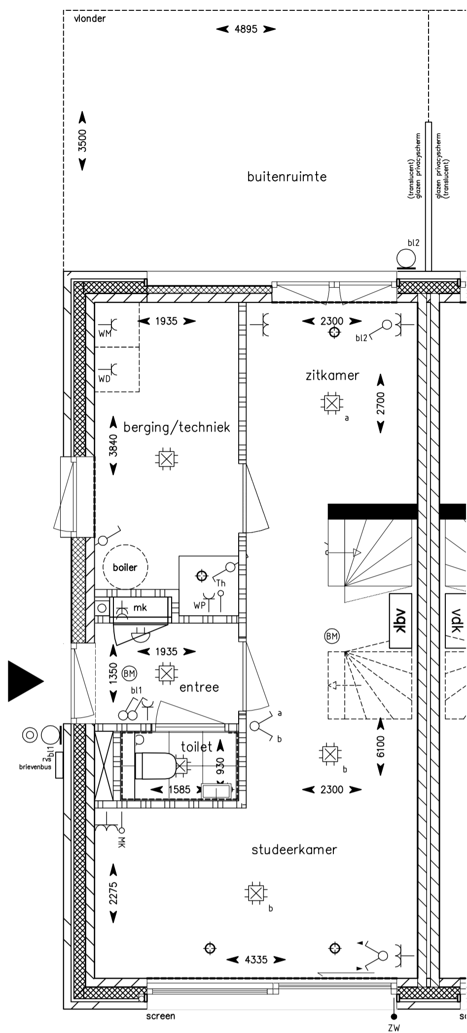
Begane grond
