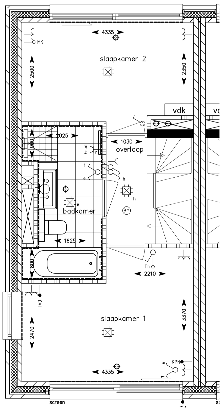
2e verdieping
