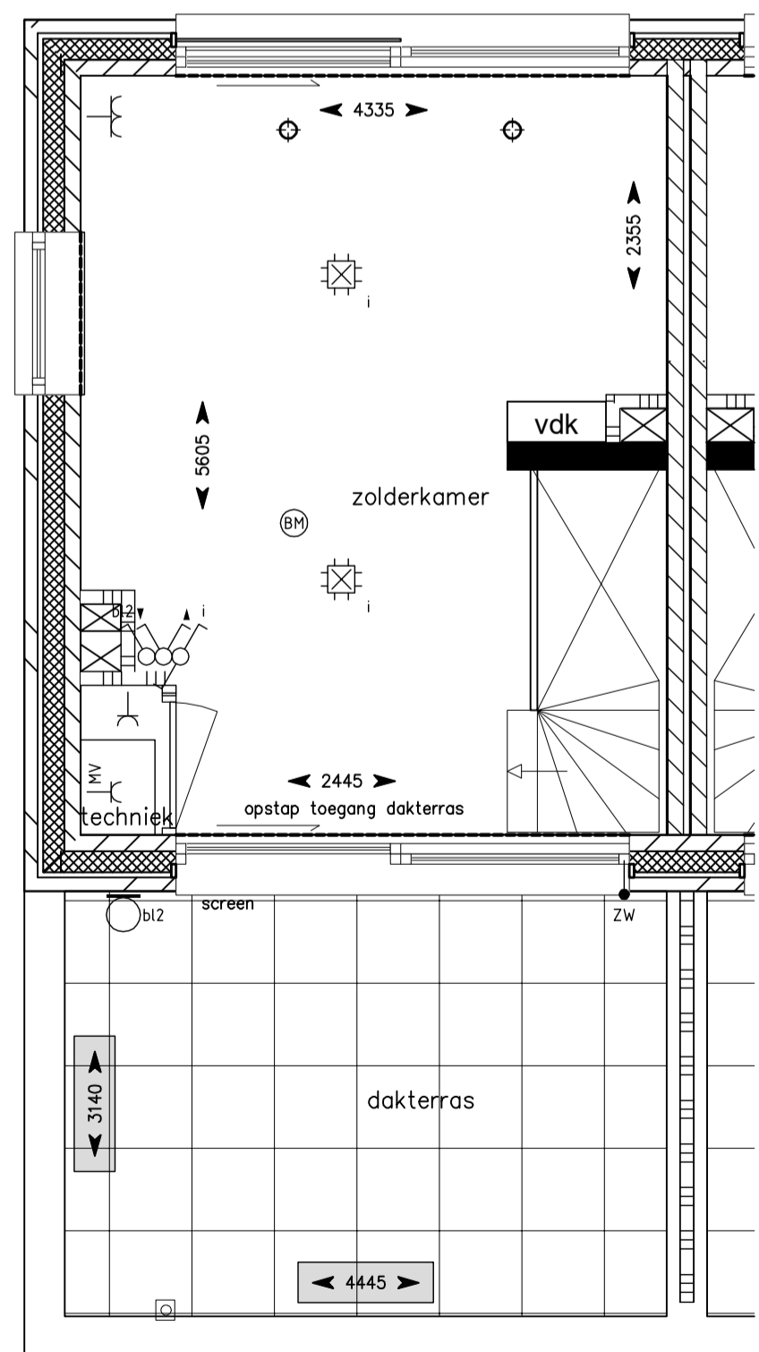
3e verdieping
