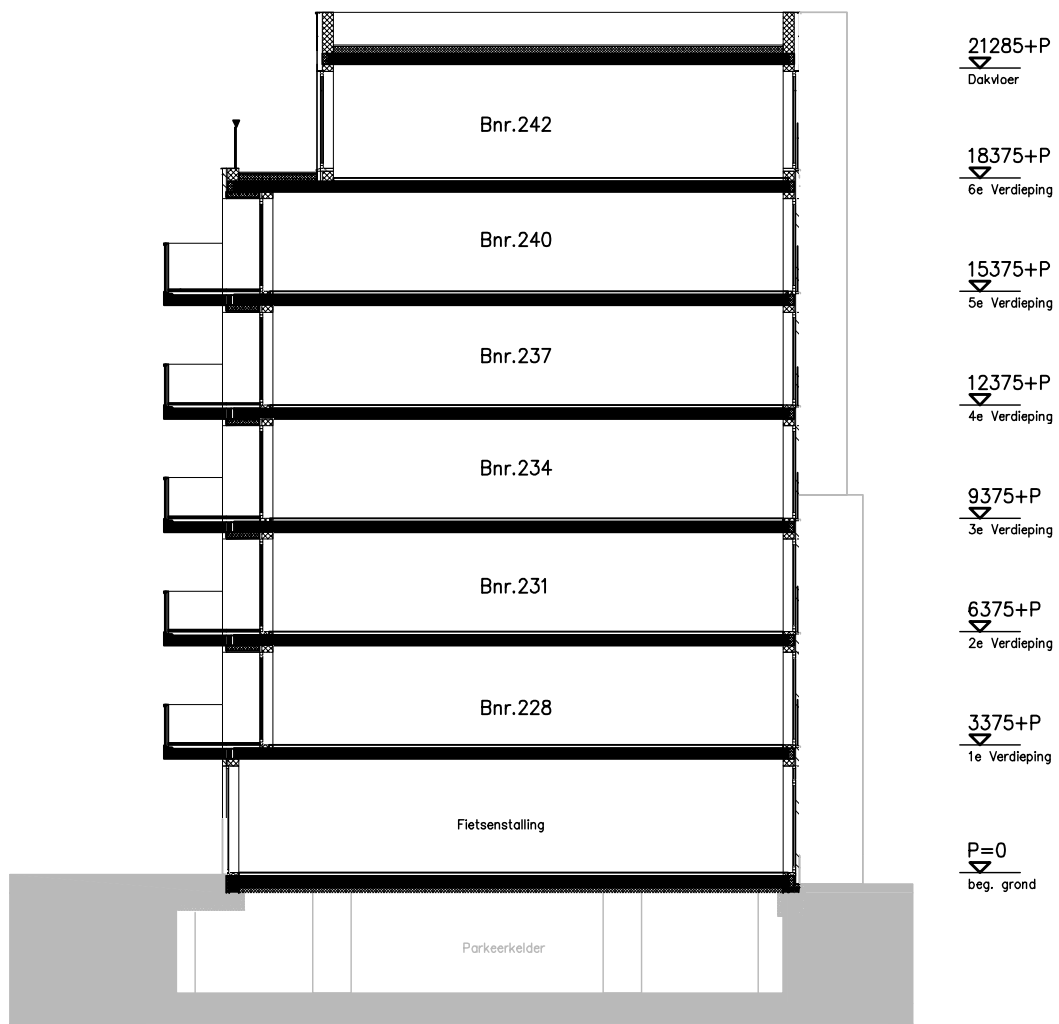
Dwarsdoorsnede 1 Blok J
