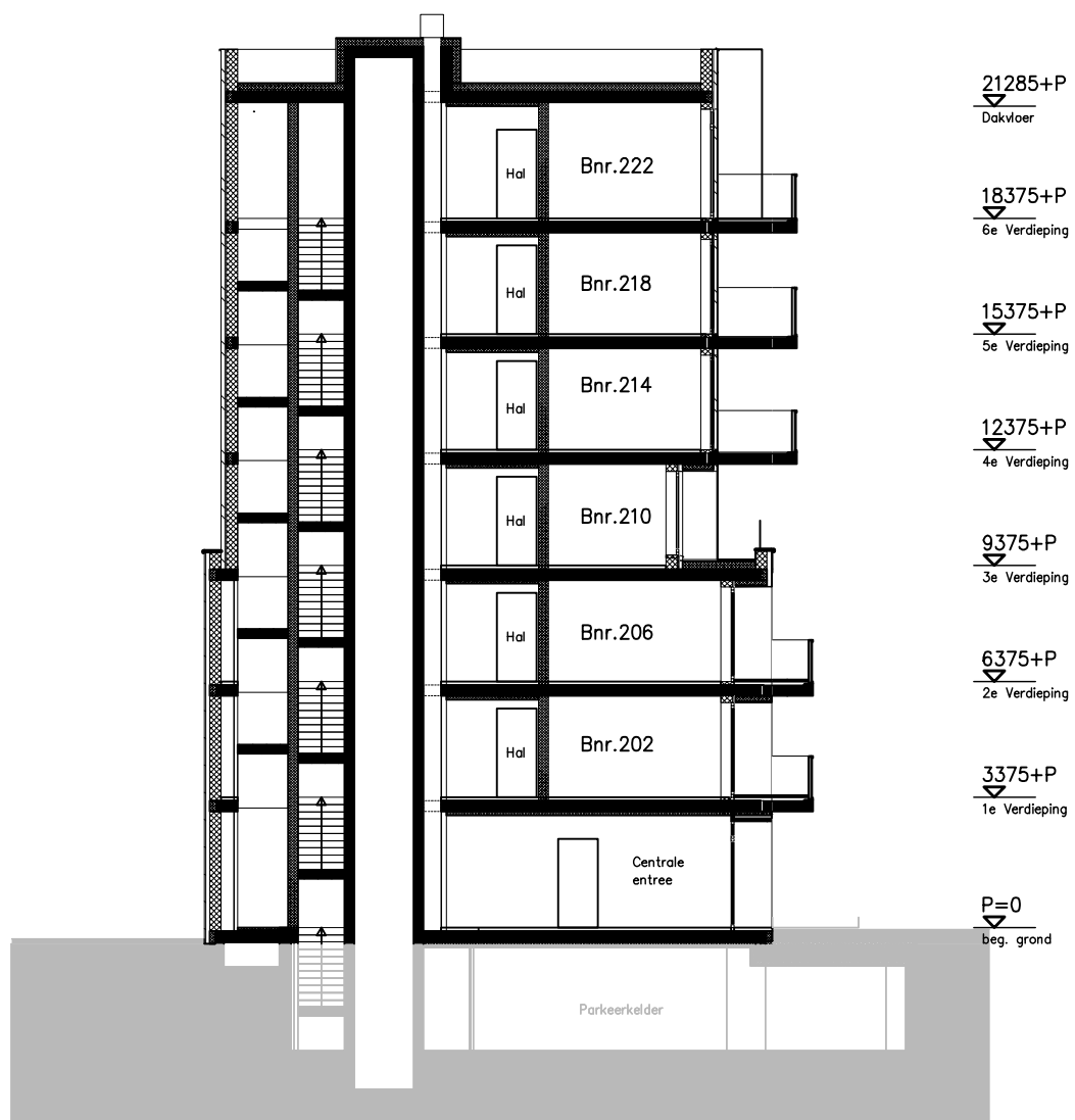
Dwarsdoorsnede 2 Blok I
