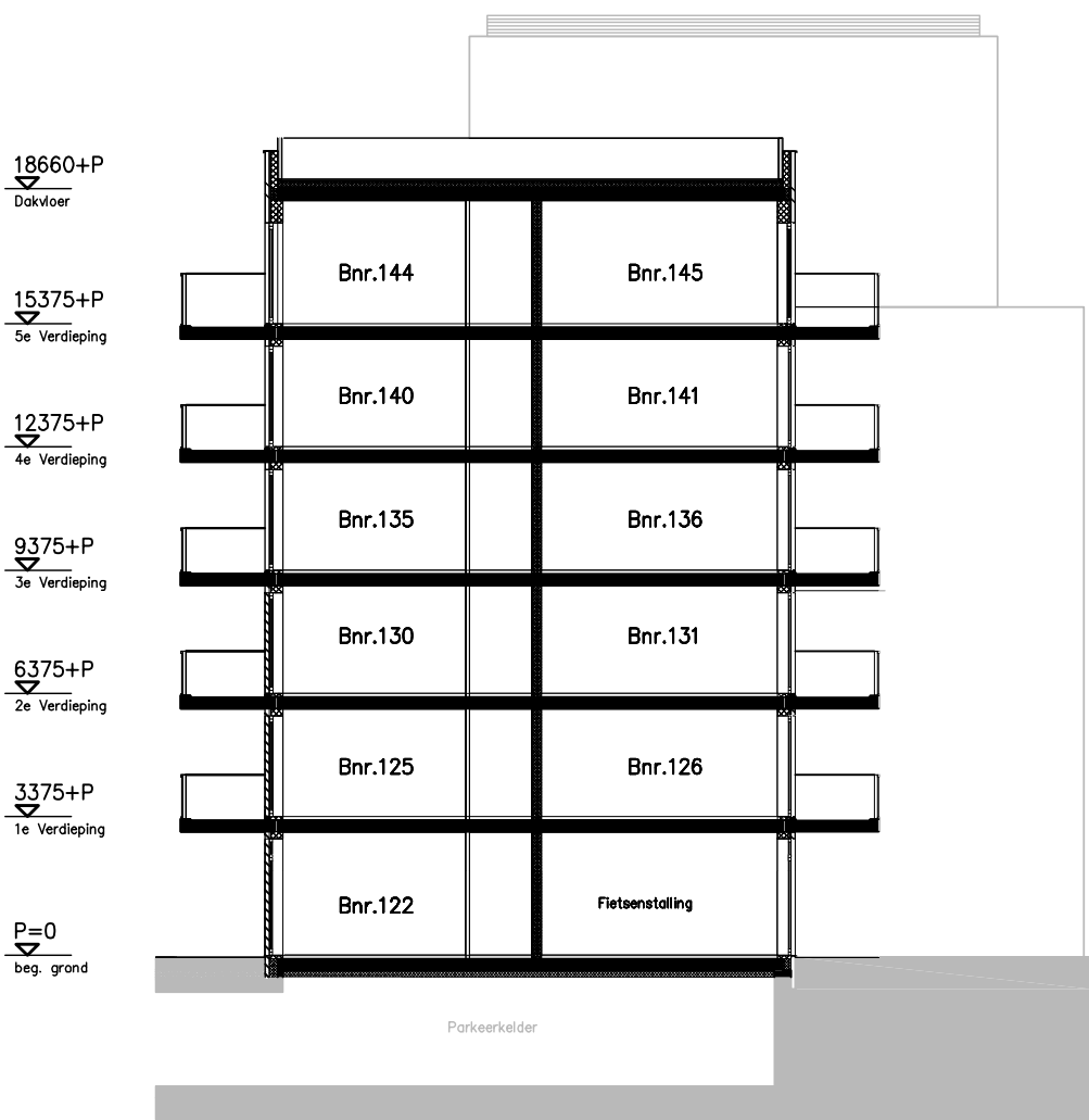
Dwarsdoorsnede Blok F
